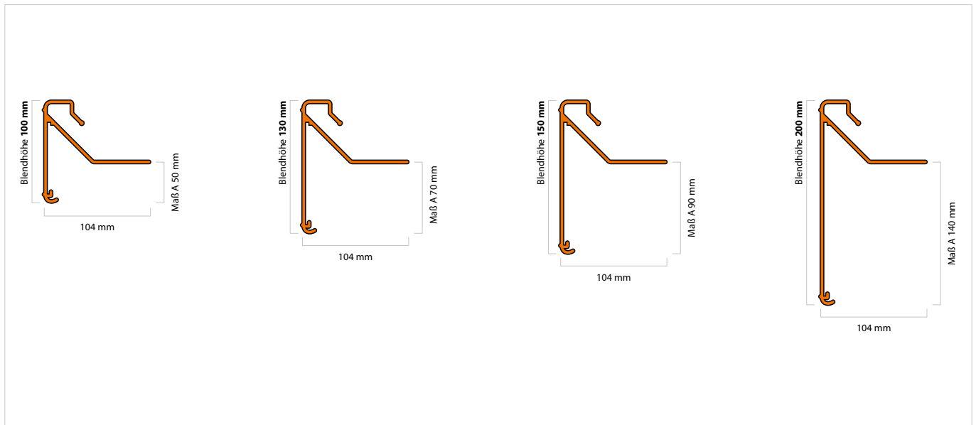
Querschnitt Solo
