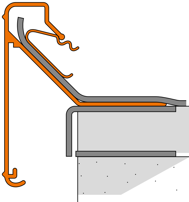
Querschnitt SOLO
