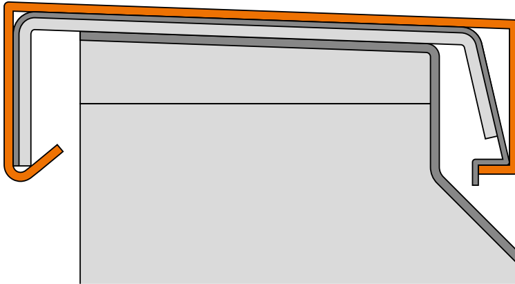
Querschnitt Mauerabdeckung
